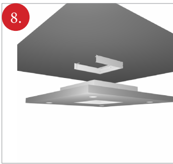
Helyezzük fel az álmennyezet sziget a mellékelt leírás szerint a LED panel rögzítő keret köré
