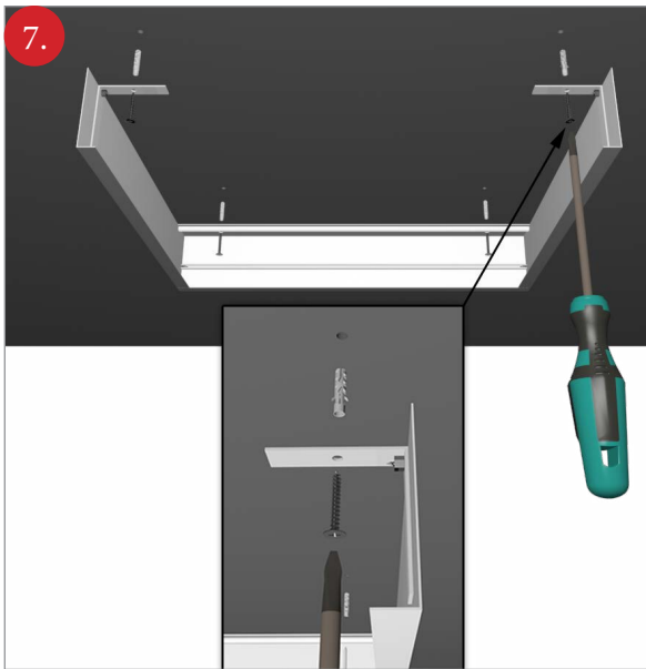
Szereljük fel a keretet, a nagyobbik csavarral, és a tiplivel
